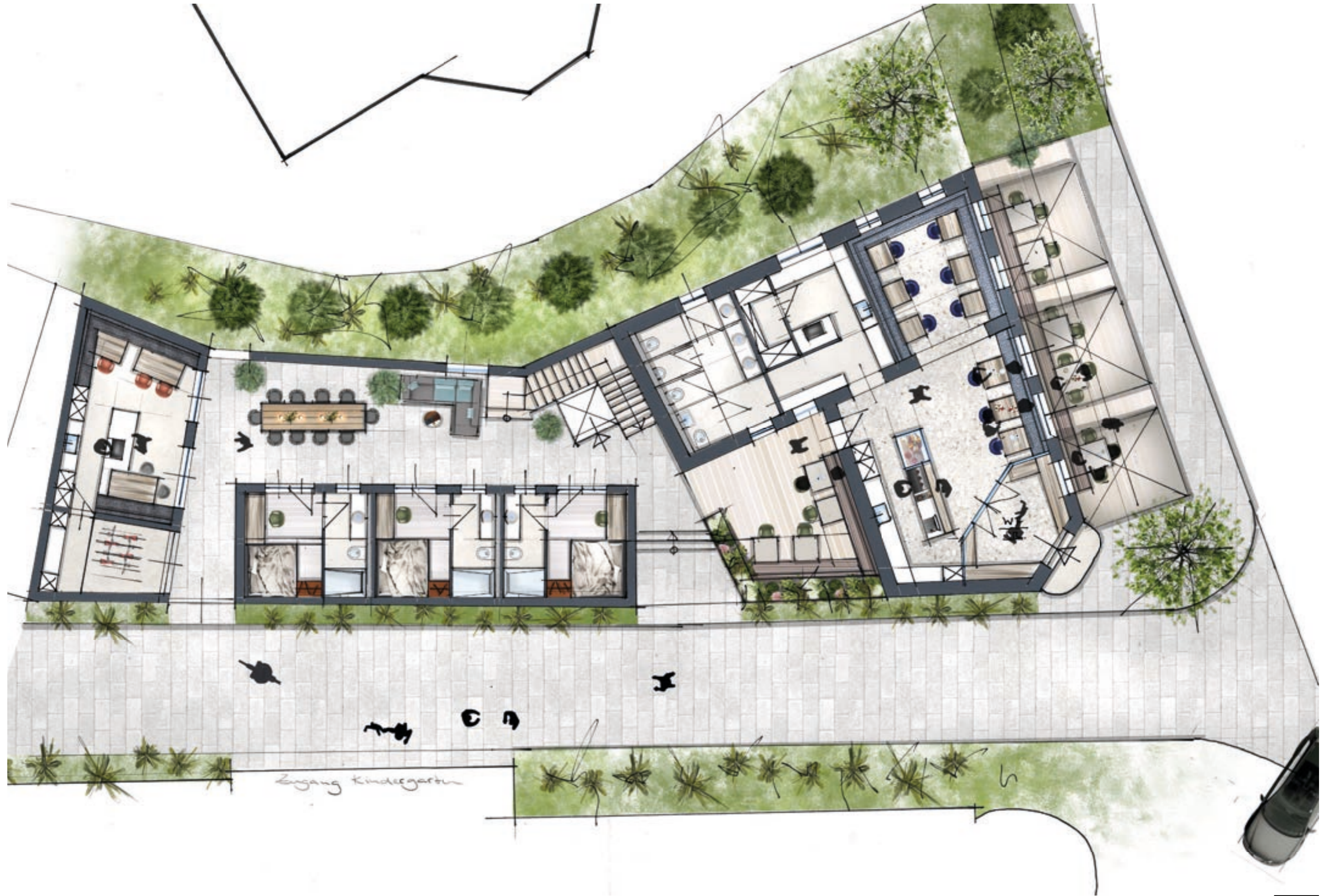
GRUNDRISS ERDGESCHOSS ÜBERSICHT OHNE MASSSTAB
